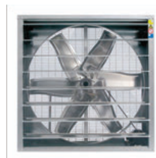
66 QUẠT HÚT CÔNG NGHIỆP BNF - 1000, 380 - 0.75KW 1000X1000X400
